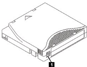
Figure 16. Positionnement du taquet de protection contre l'écriture
