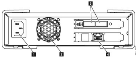
Figure 6. Panneau arrière du lecteur de bande SAS externe
