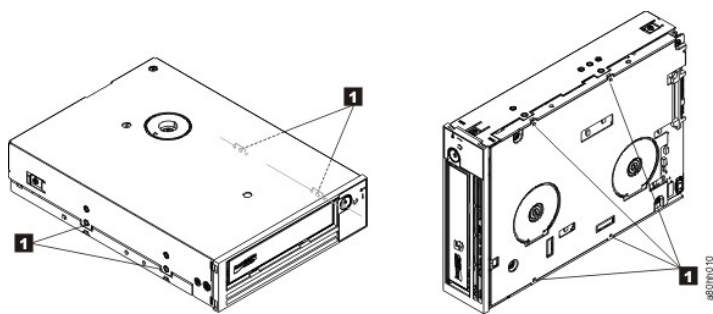
Figure 8. Trous de vis du lecteur de bande
