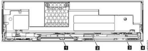
Figure 5. Panneau arrière du lecteur de bande SAS interne
